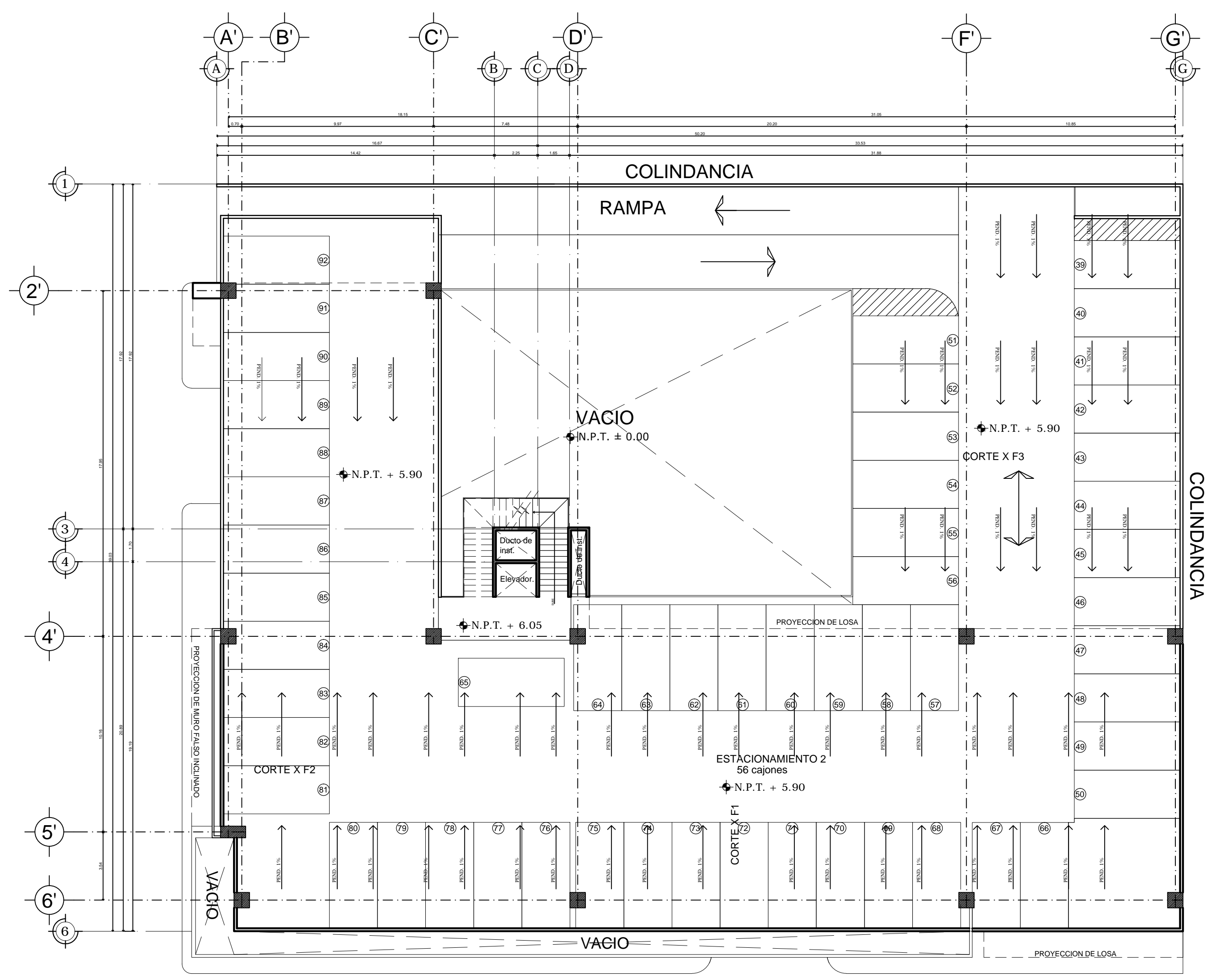
PRIMER PISO
